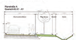
Straßenquerschnitt, Waack + Dähn
