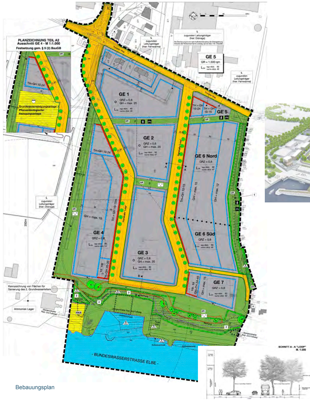
Masterplan me di um
